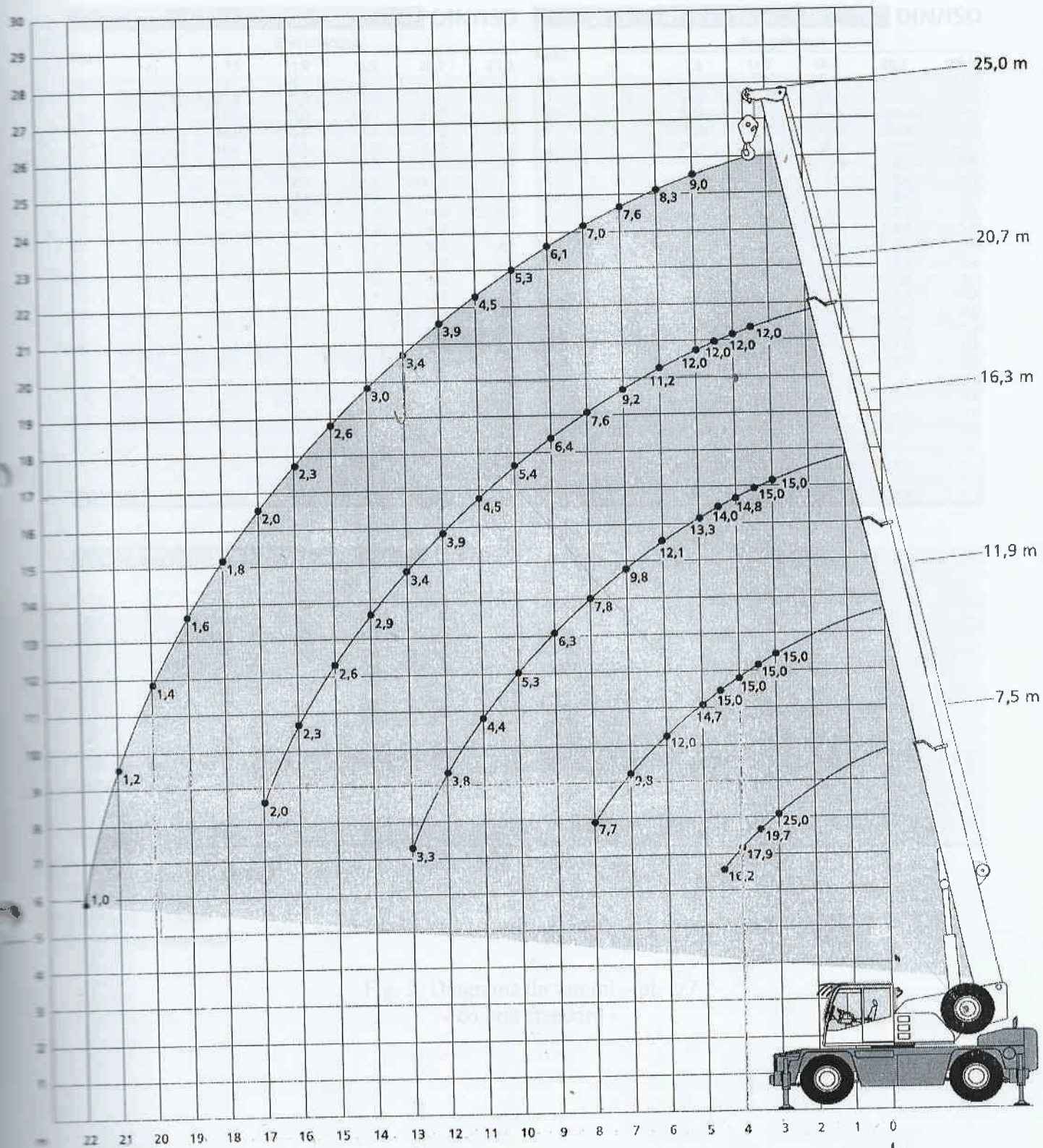
Fig. 2. Diagrama de sarcini – pl.1/7 - cu braț standard -
