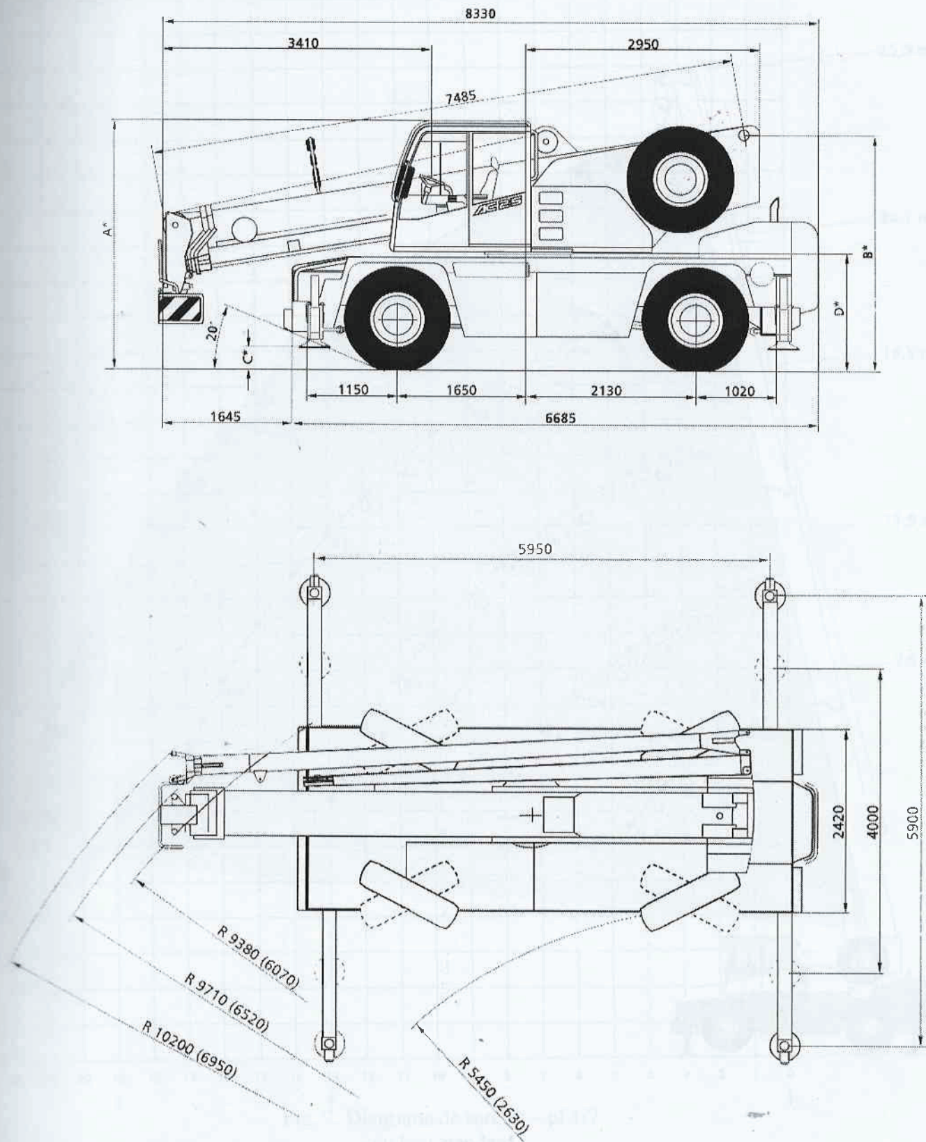
Fig. 1. Dimensiuni de gabarit
